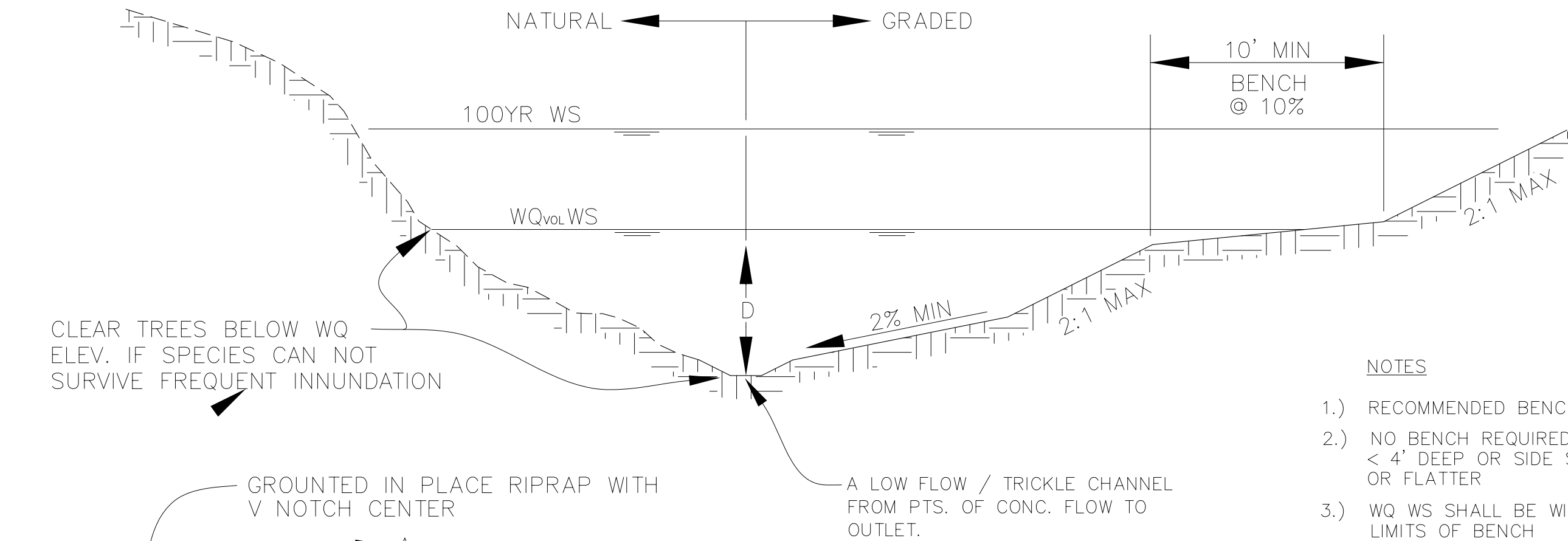
SECTION A-A
