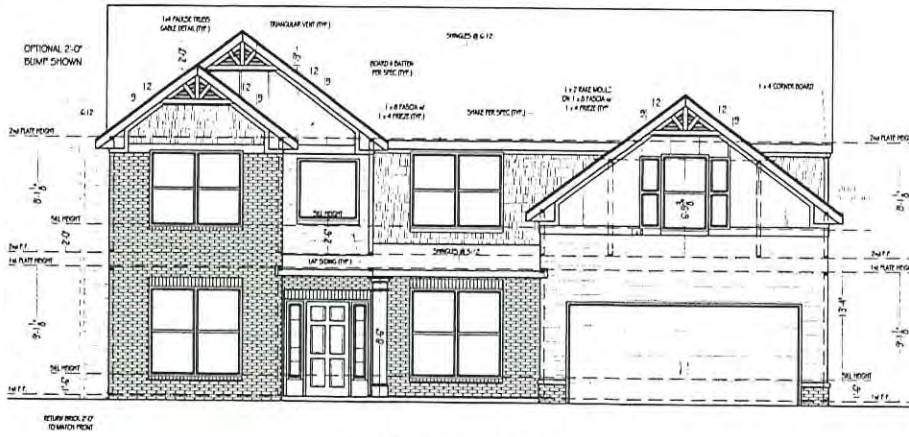
FRONT ELEVATION F3 SCALE: 1/8" = 1'-0"
